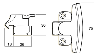
Non lockable
